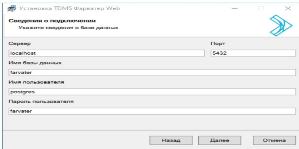
Рис. 6. Окно заполнения реквизитов для подключения к базе данных
