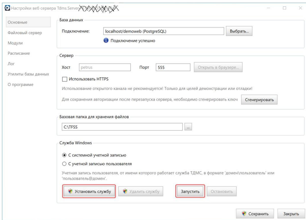
Рис. 19. TDMS Фарватер Web Конфигуратор. Кнопки установки и запуска службы
