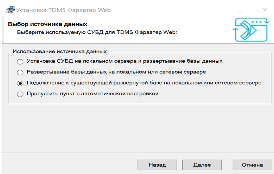
Рис. 10. Окно выбора источника данных. Подключение к базе данных на ранее установленной СУБД
