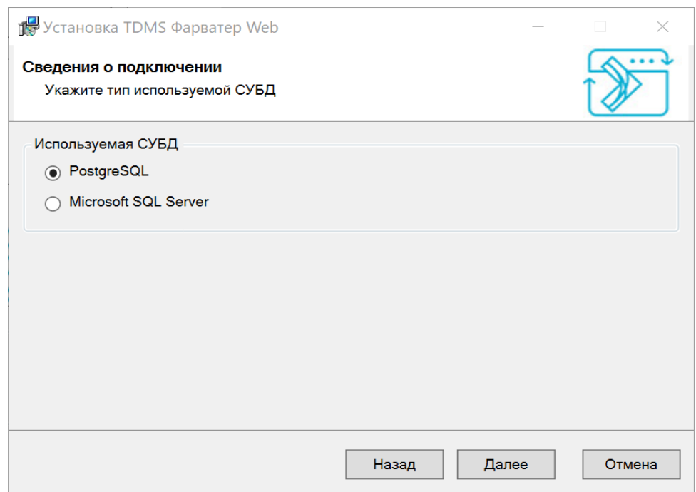
Рис. 8. Выбор типа СУБД
