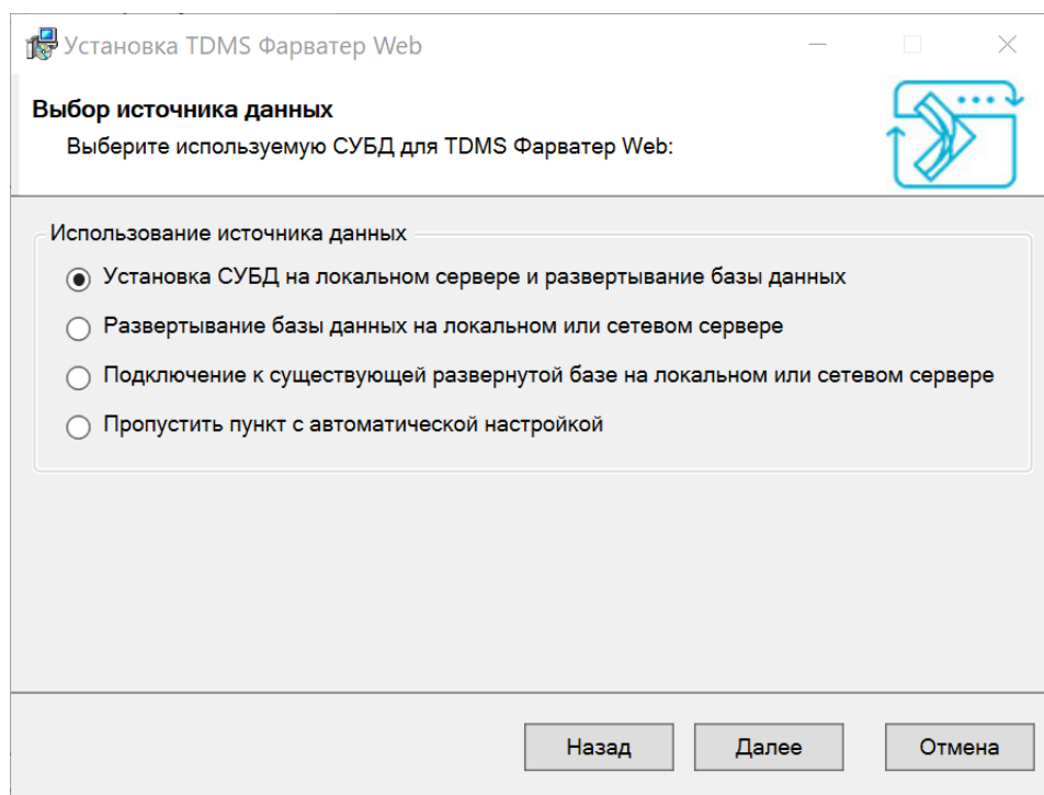
Рис. 5. Окно выбора источника данных. Вариант «Установка СУБД и развертывание базы данных»
